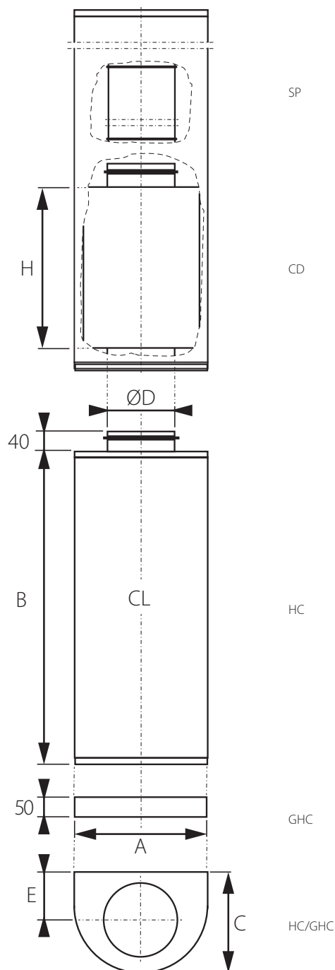
Bild 1. Mått (mm), luftdon HC med tillbehör, sockel GHC, inklädnad IHC *) . Ljuddämpare CD och spjäll märkt SP, innanför inklädnaden.
