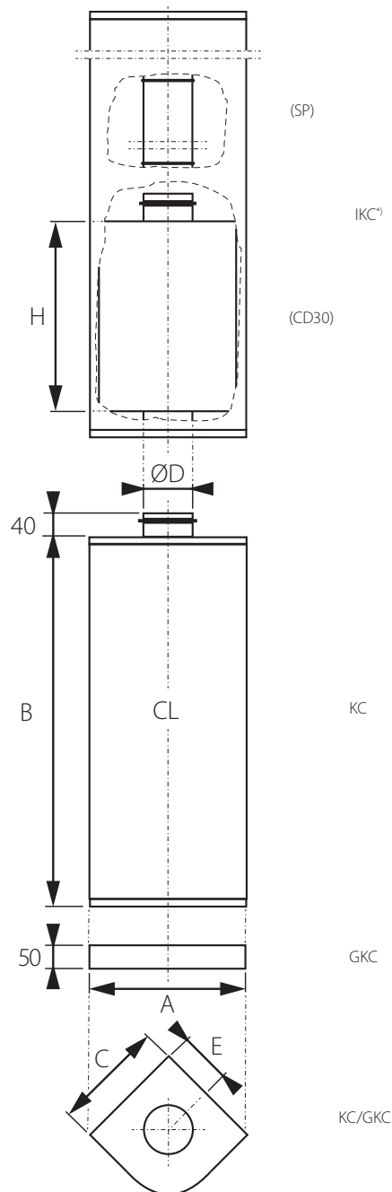
Bild 1. Mått (mm), luftdon KC med tillbehör, sockel GKC, inklädnad IKC*). Ljuddämpare CD30 och spjäll märkt SP, innanför inklädnaden.
