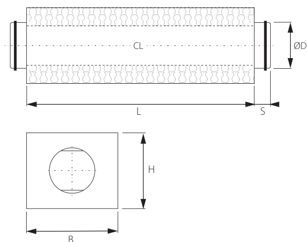
Bild 1. Mått, ljuddämpare C-LÅG.
