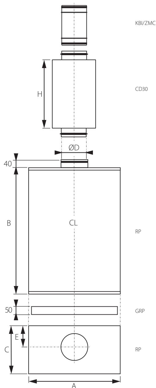
Bild 1. Mått, luftdon RP, version a med tillbehör sockel GRP, ljuddämpare CD30 samt spjäll märkt SP (mm).
