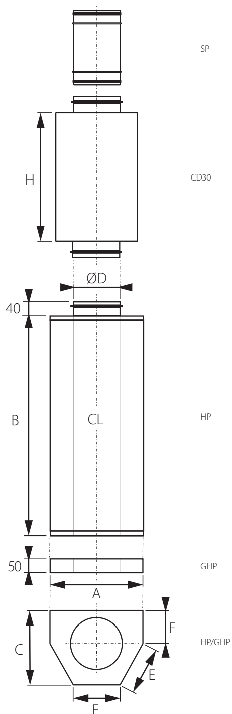
Bild 1. Mått, luftdon HP med tillbehör sockel GHP, ljuddämpare CD30 samt spjäll märkt SP (mm).
