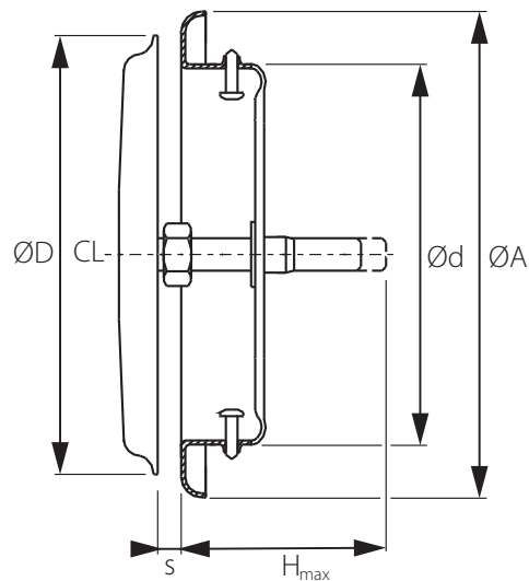
Bild 1. Mått, tallriksventil VT.
