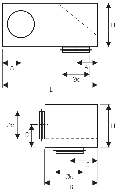
Bild 1. Mått, ljuddämpare CU.
