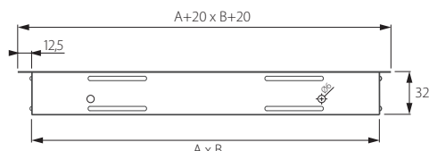
Bild 1. Mått (mm), fästram RAM.
