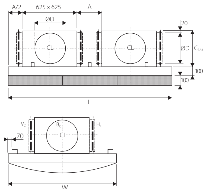
Bild 2. Mått, MHOS (mm).
