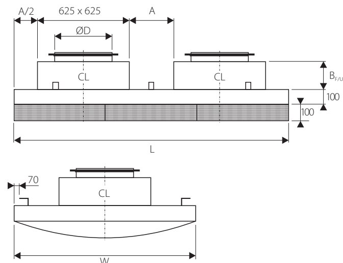
Bild 1. Mått, MHO (mm).
